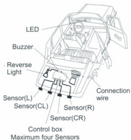
Obr. 2 - Umístění jednotlivých částí parkovacího systému
