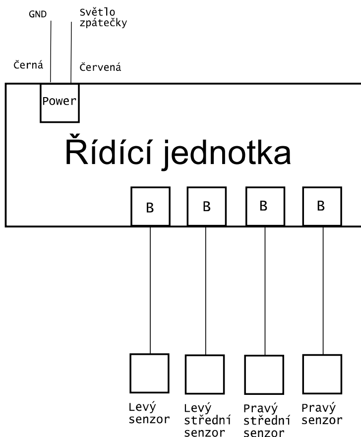
Obr. 7 – Schéma zapojení parkovacího systému.
