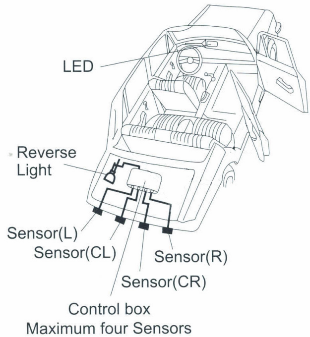
Obr. 2 - Umístění jednotlivých částí parkovacího systému
