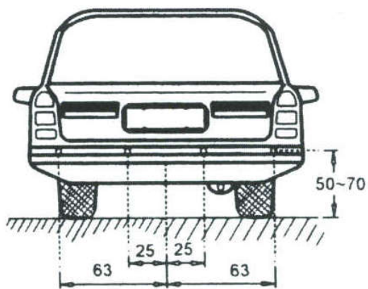
Obr. 3 - Umístění senzorů na zadním (u PLC-85 i předním) nárazníku, hodnoty jsou v cm
