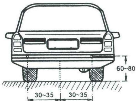
Obr. 4 - Umístění senzorů na předním nárazníku (PLC-65), hodnoty jsou v cm
