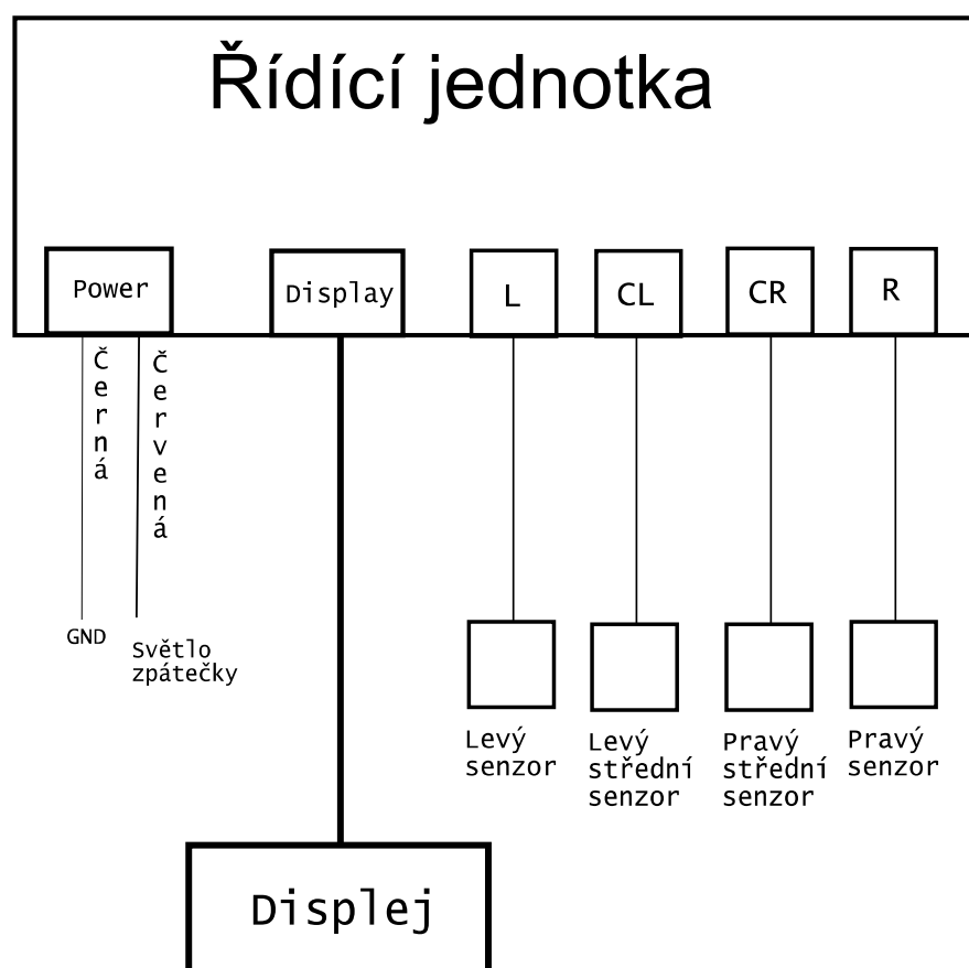
Obr. 7 – Schéma zapojení parkovacího systému.
