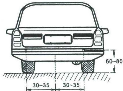
Obr. 5 - Umístění senzorů na nárazníku (2 senzory), hodnoty jsou v cm
