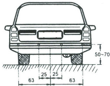
Obr. 4 - Umístění senzorů na nárazníku (4 senzory), hodnoty jsou v cm
