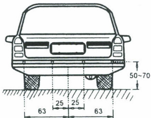
Obr. 4 - Umístění senzorů na zadním nárazníku (pro PWM-84 i na předním nárazníku), hodnoty jsou v cm
