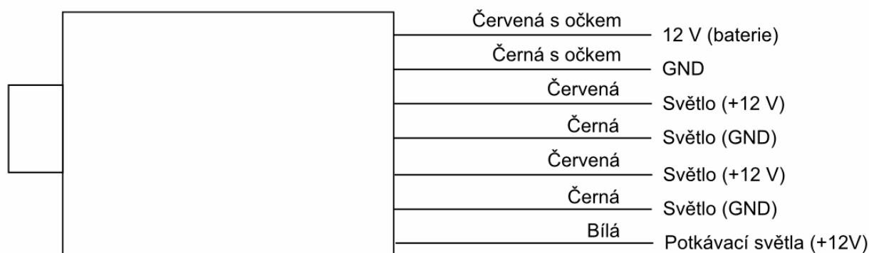
Obrázek 1: Schéma zapojení
